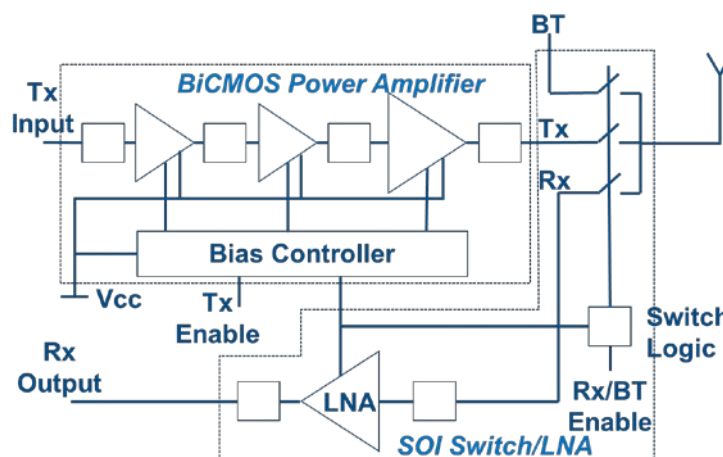
Fig. 7: 2GHz WLAN Front-end Module [2]
