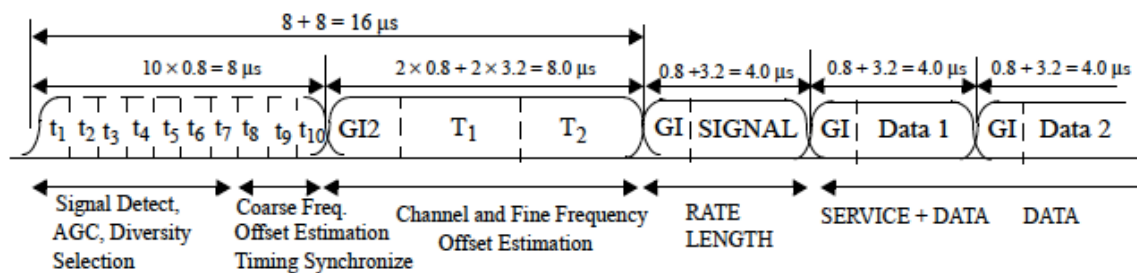
Fig. 5: 802.11a Frame
